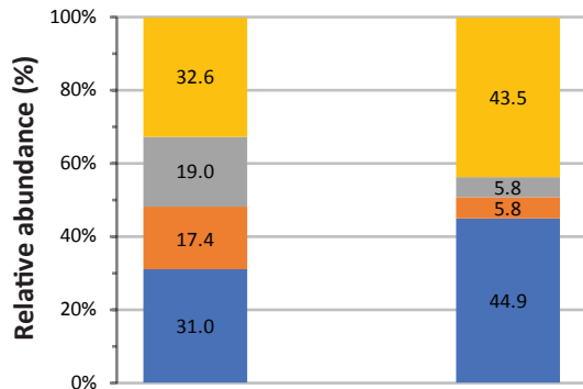
S. microadriaticum (A1)
