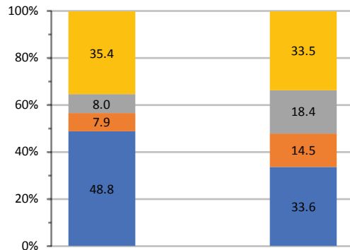
B. minutum (B1)
