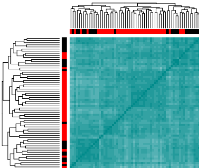
Colon – Ochiai, J=2
