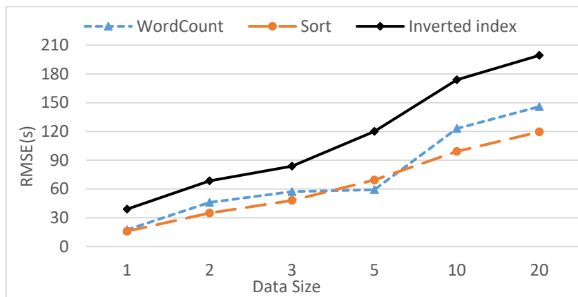
Fig. 7 – RMSE values
