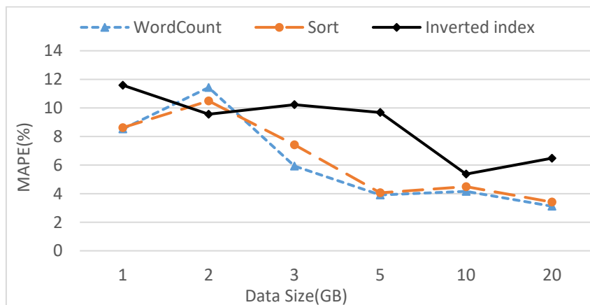
Fig. 8 – MAPE values
